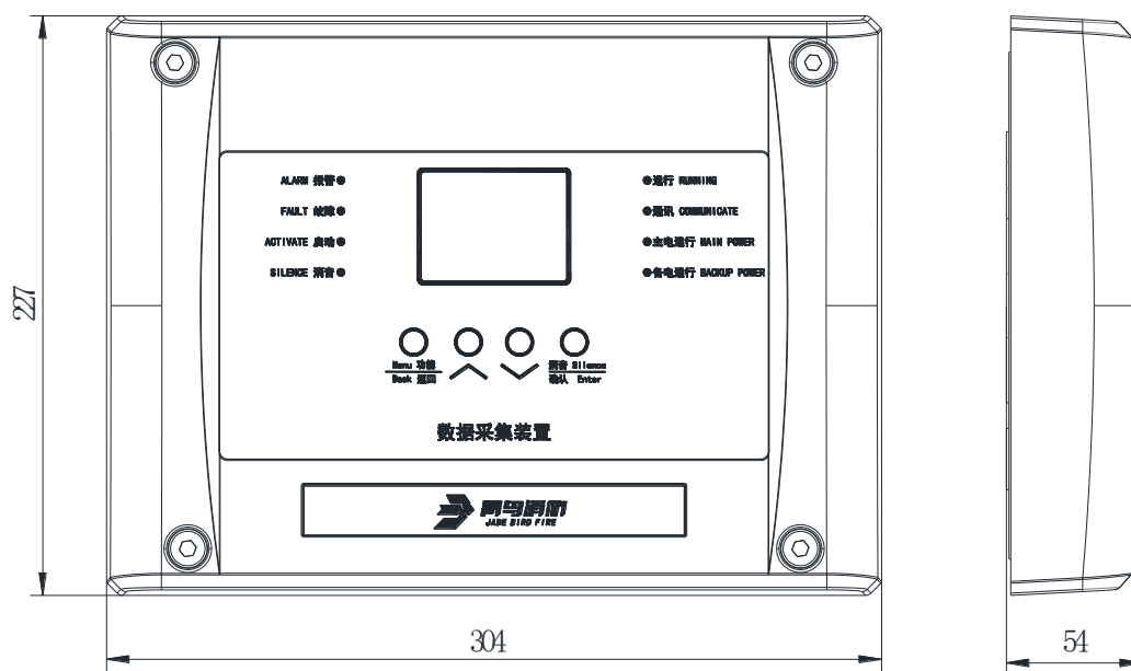
图 1 外形尺寸图
