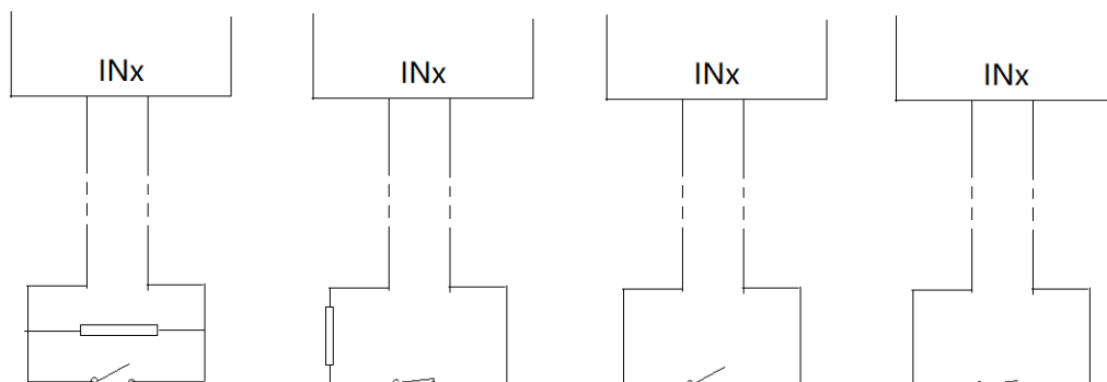
图 47 输入端口接线
