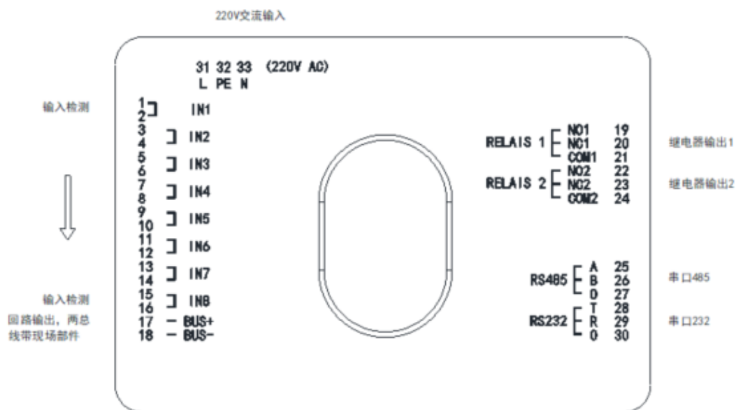
图 3 端子接线图
